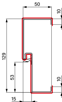
OŚCIEŻNICA STALOWA
