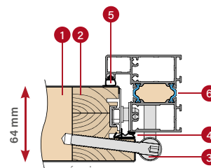
OŚCIEŻNICA ALUMINIOWA
