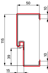
OŚCIEŻNICA STALOWA
