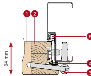
OŚCIEŻNICA STALOWA
